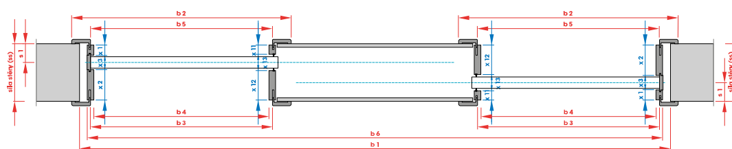
Jednokřídlé UNIBOX šířka/výška (mm)
