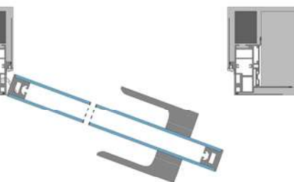
Dveře otočné jednokřídlé levé
