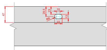
ZÁRUBEŇ PRAVÁ
