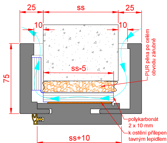
bezpoldrážková SAPGLASS s provětráváním ( ss_{\min.} = 80 \text{ mm} )
