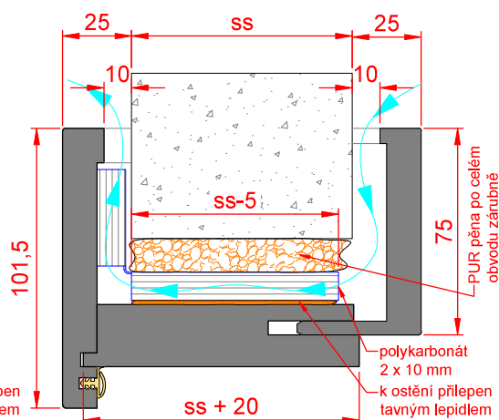
reverzní s provětráváním ( ss_{\min.} = 80 \text{ mm} )
