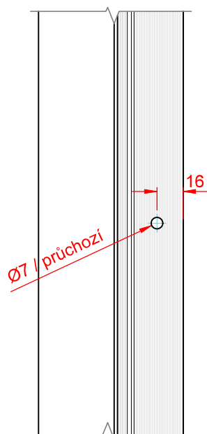
detail "A" (vrtání pro RC kotvu)
