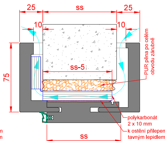
polodrážková s provětráváním ( ss_{\min.} = 80 \text{ mm} )
