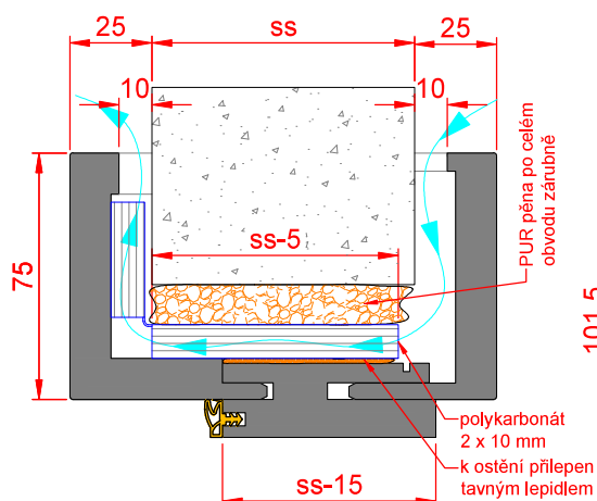
bezpoldrážková s provětráváním ( ss_{\min.} = 80 \text{ mm} )
