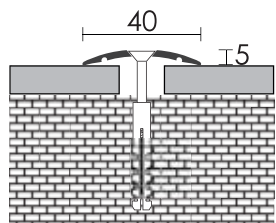
Přechodová lišta vrtaná, hliník
