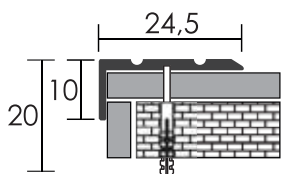
Pravouhlý schodový profil - vrtaný, hliník
