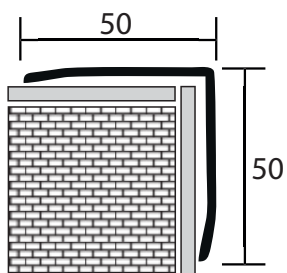
Pravoúhlý profil nerez
