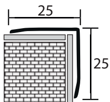
Pravoúhlý profil nerez
