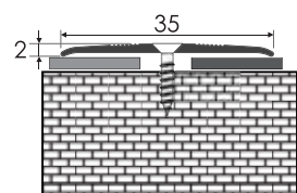
Přechodová lišta plochá vrtaná, hliník
