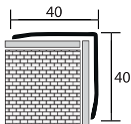
Pravoúhlý profil nerez
