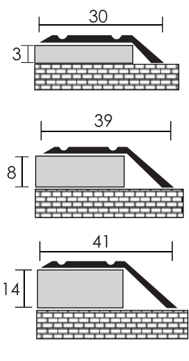
Ukončovací profil samolepící, hliník
