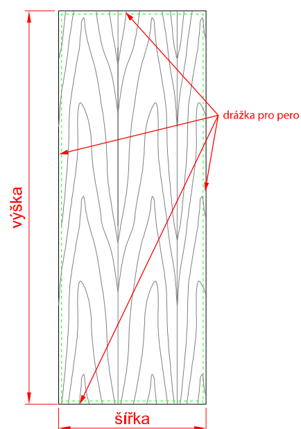
OBKLADOVÝ PANEL LPHS
