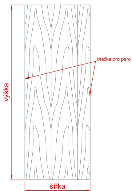
OBKLADOVÝ PANEL LP
