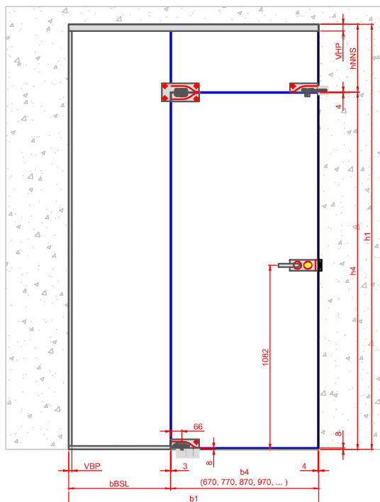
Model T Jednokřídlé Kynné Levé
