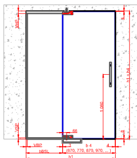
Model B Jednokřídlé Kynné Levé
