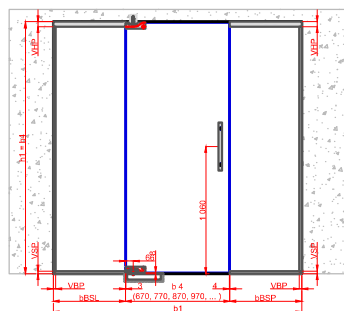
Model C Jednokřídlé Kynné Levé
