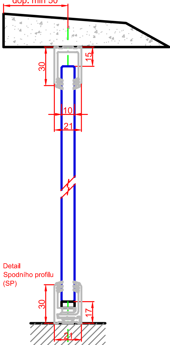
Detail Horního profilu (HP) dop. min 50
