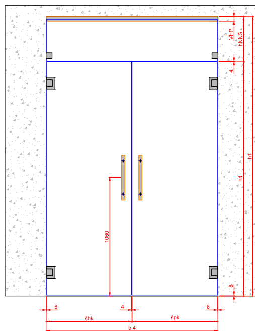
Model A Dvoukřídlé Kyvné + Kyvné Levé
