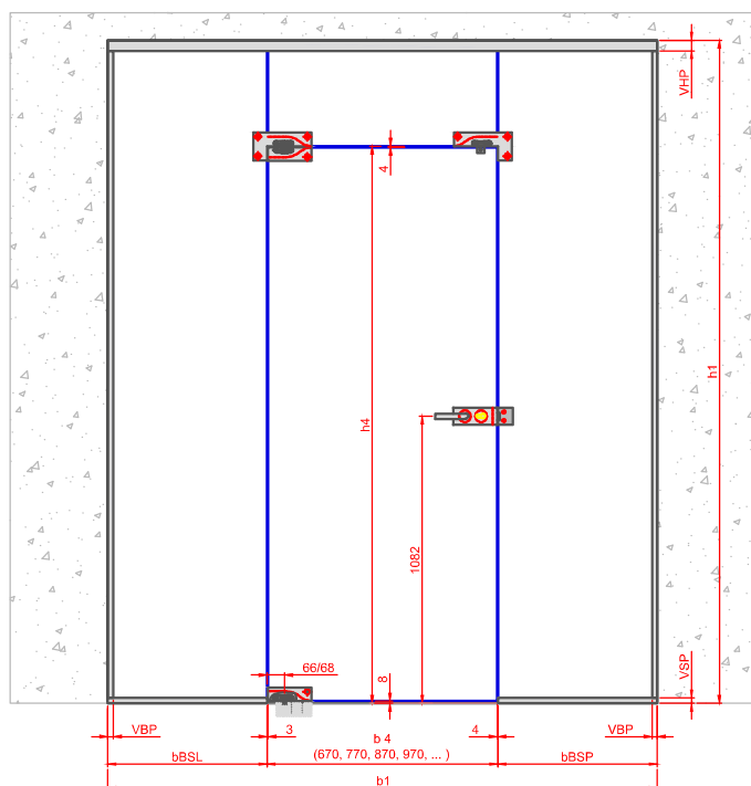
Model U Jednokřídlé Kyvné Levé
