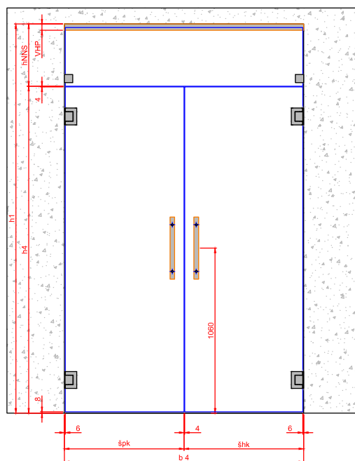
Model A Dvoukřídlé Kyvné + Kyvné Pravé
