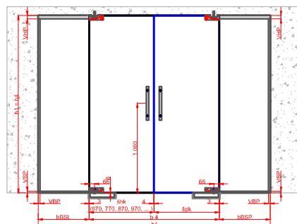
Model C Dvoukřídlé Kynné + Kynné Levé
