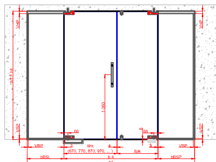
Model C Dvoukřídlé Kynné + Pasivní Levé
