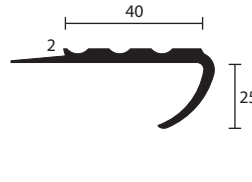
Položka 13385 TK 40/25/2
