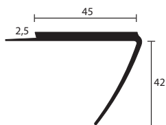
Položka 13389 TK 45/42/2,5
