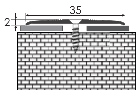
Přechodová lišta plochá vrтанá, hliník
