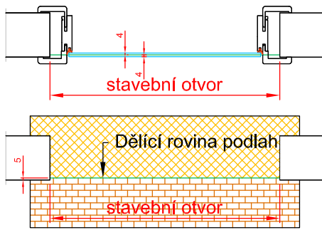
Zárubeň polodrážková Normal, Obtus, Dveře otočné SAPGLASS
