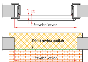
Dveře otočné polodrážkové
