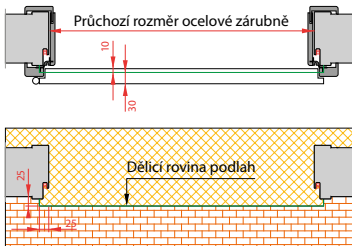
Dveře otočné polodrážkové se zárubní OKZ
