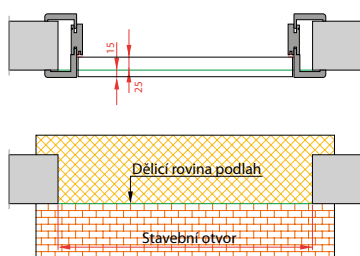
Dveře otočné bezpolodrážkové
