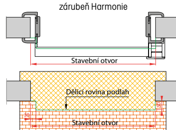
Dveře jednokřídlé posuvné na stěnu – zárubeň Harmonie
