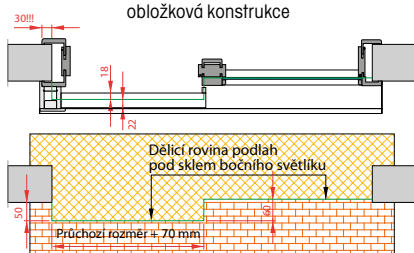
Dveře posuvné s bočním světlíkem – obložková konstrukce
