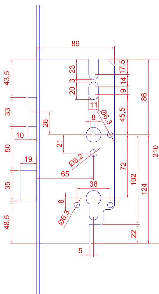
zámek GENIUS KVV AS2602 CA, CB (2600_1)
