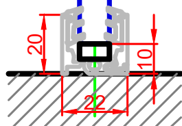
Detail Spodního profilu (SP)
