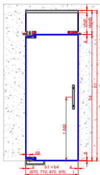
Model A Jednokřídlé Kynné Levé
