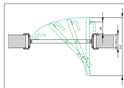
Výpočet prostoru pro kliku PK (mm):
