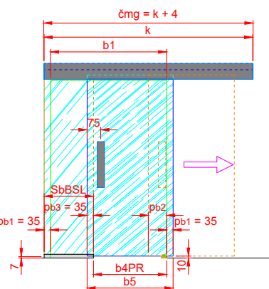
model B 1K - křídlo pravé (model K - křídlo levé => zrcadlořev)
