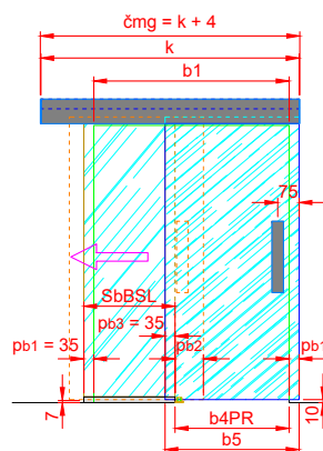
model B 1K - křídlo levé (model K - křídlo pravé => zrcadlořev)
