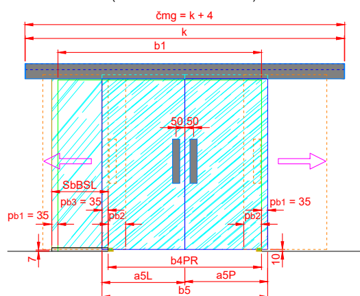
model B 2K (model K 2K => zrcadlořev)
