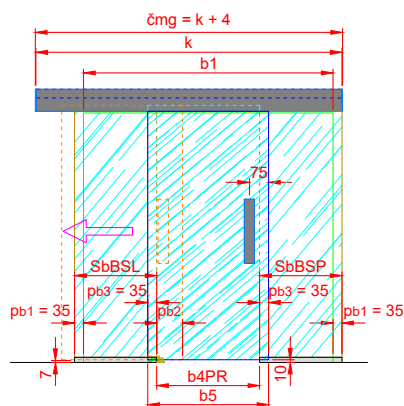
model C 1K - křídlo levé (křídlo pravé zrcadlořev)
