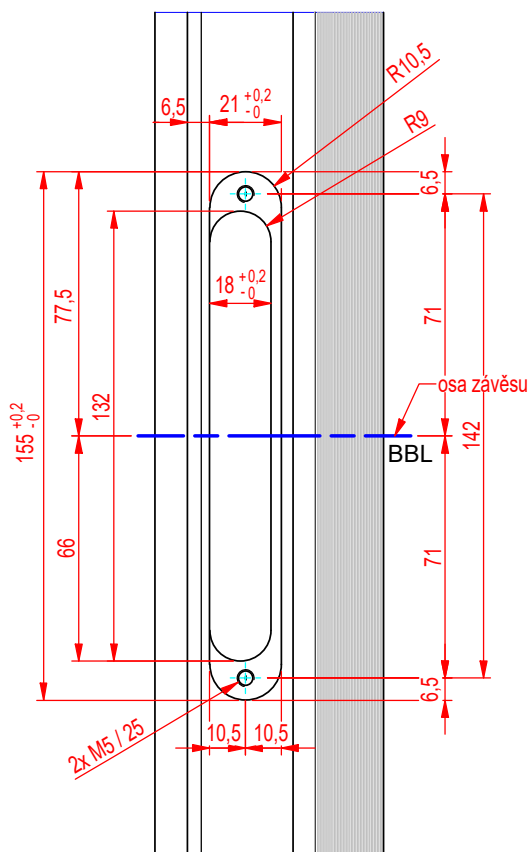
detail A ( 1 : 2 )
