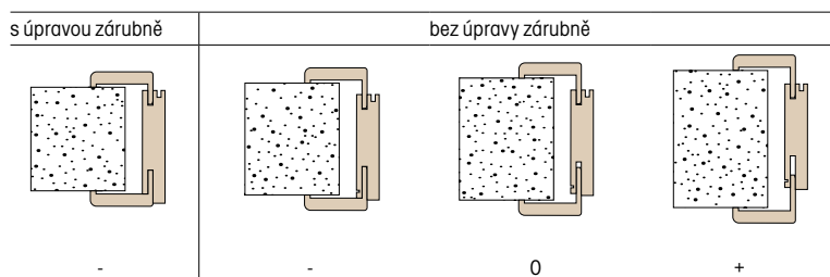
Regulace zárubní
